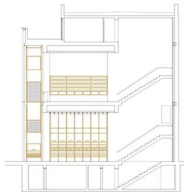
SCHNITT (LINKS)
