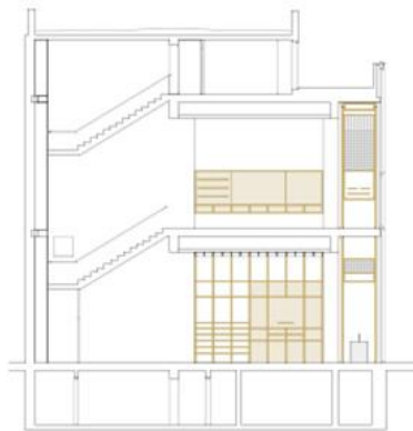
SCHNITT (RECHTS)
