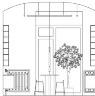
Pohled C
