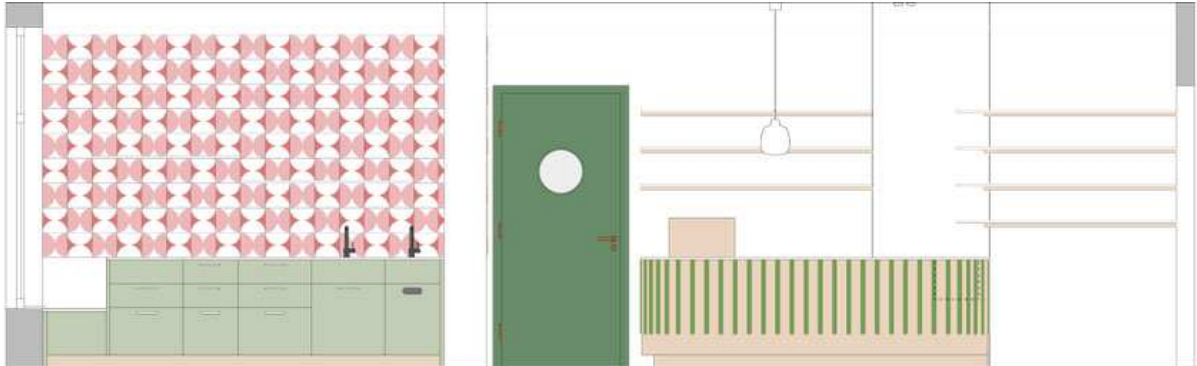
Ansicht Kassentheke, Schauproduktion
